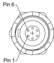
Anschlussbuchse – Pinbelegung (Vorderansicht)
