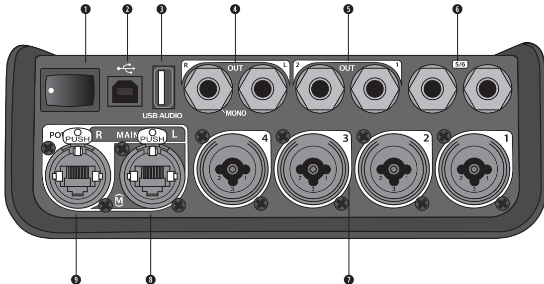
Abbildung 2. T4S Anschlussleiste
