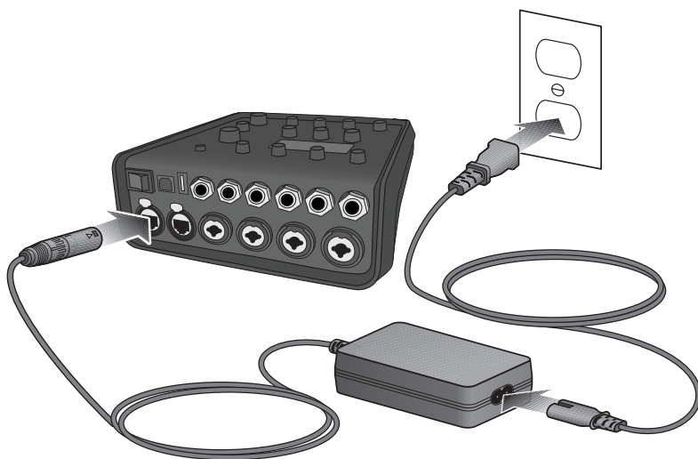
Figura 11 Collegamento del mixer T4S all'alimentatore
