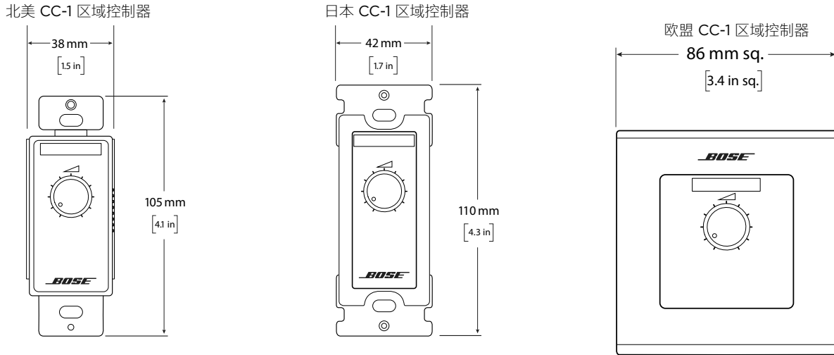
图 7.CC-1 ControlCenter 区域控制器
