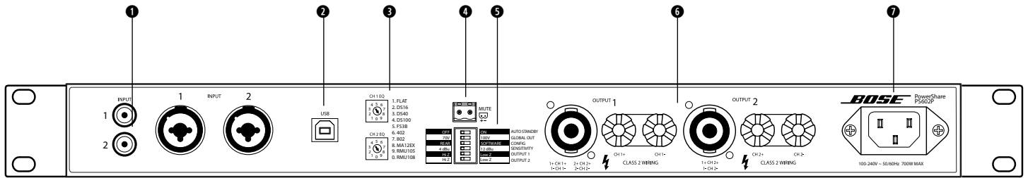
图 5. PowerShare PS602P 功放后面板
