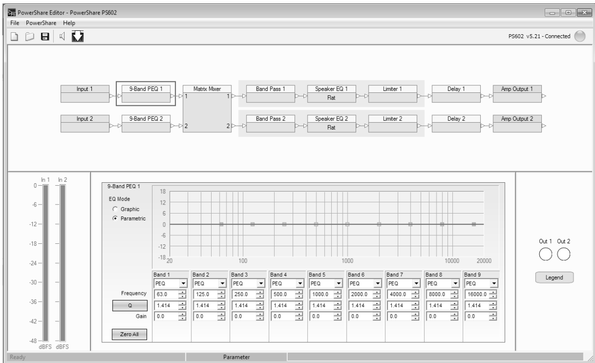
图 10.PowerShare Editor 软件上有关 PS602 和 PS602P 功放的双通道配置
