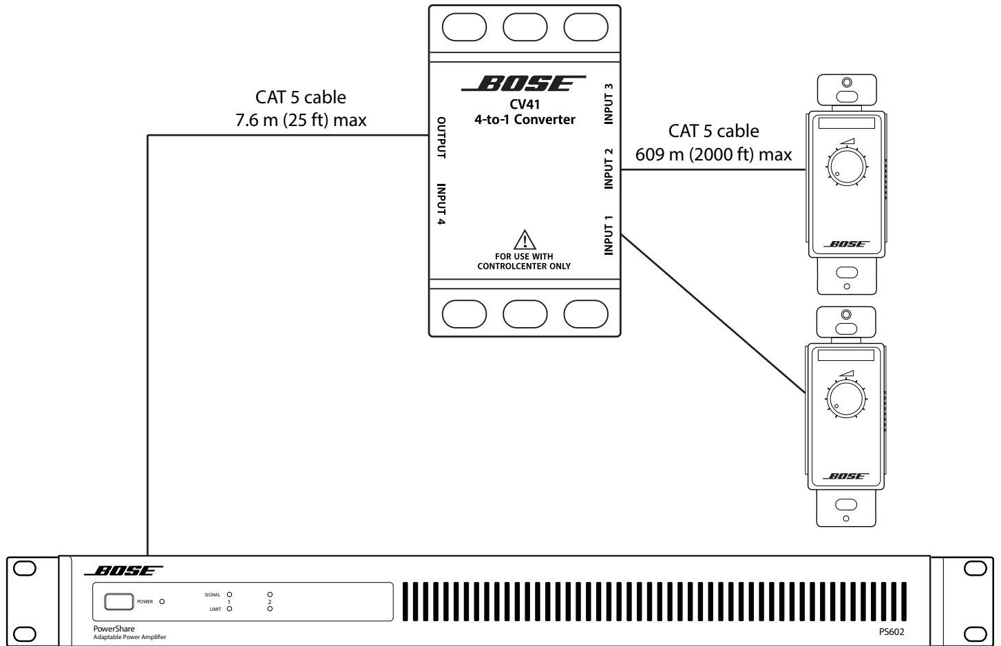
图 9. 分布式 CC-1 ControlCenter 区域控制器连接至功放
