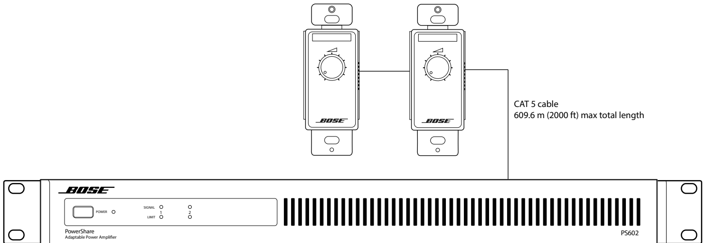
图 8.直接式 CC-1 ControlCenter 区域控制器连接至功放
