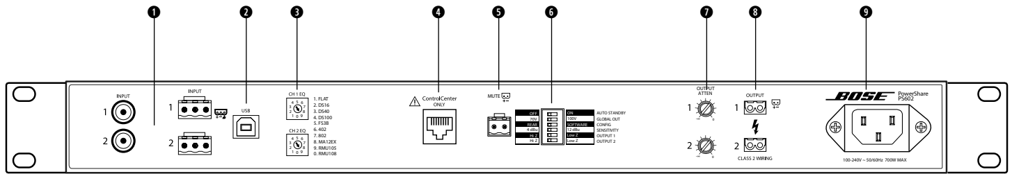
图 3. PowerShare PS602 功放后面板
