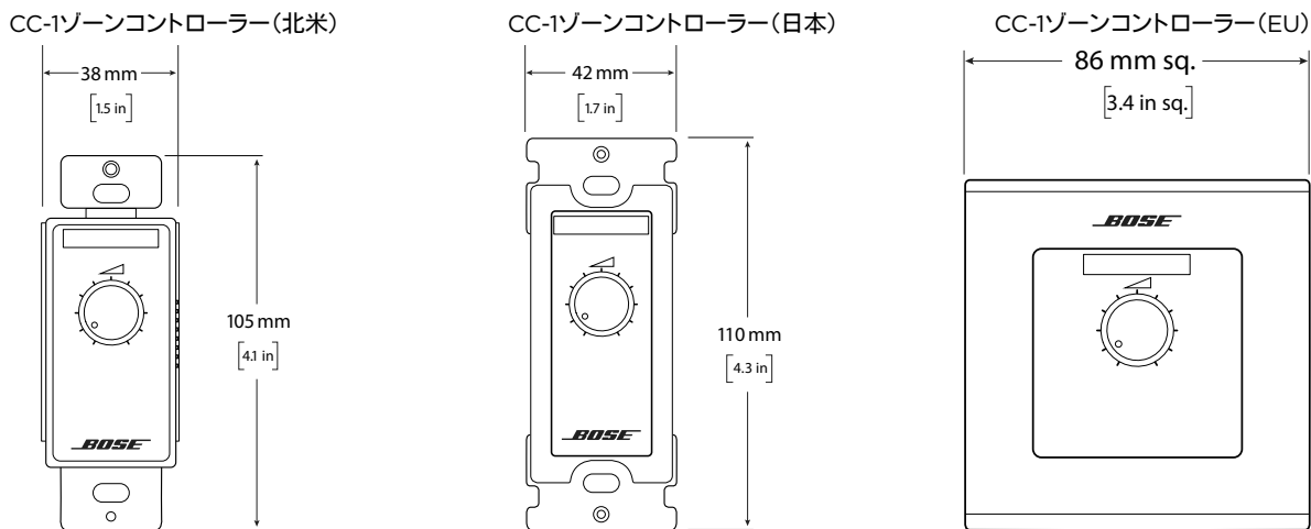
図5.CC-1 ControlCenterゾーンコントローラー
