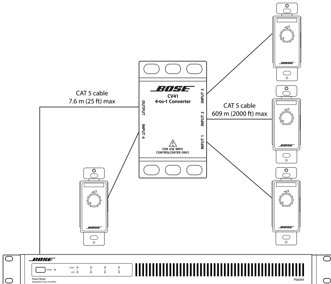
図7.CC-1 ControlCenterゾーンコントローラーのアンプへの接続 - 分散接続する場合
