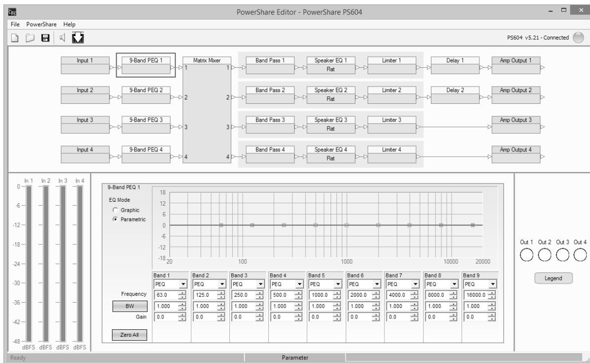
図8.PS604AおよびPS404AアンプのPowerShare Editorソフトウェアコンフィギュレーション画面
