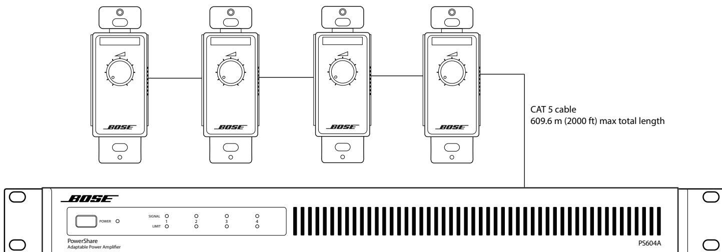
図6.CC-1ゾーンコントローラーのアンプへの接続 - 直接接続する場合
