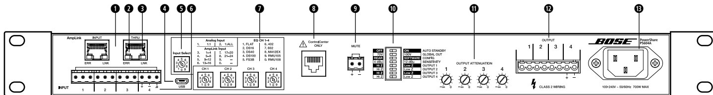
図3.PowerShare PS604Aアンプのリアパネル
