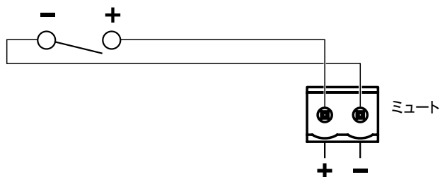
図4.アンプのミュートコンタクトクローザー
