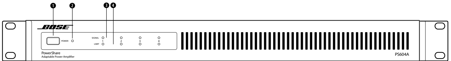
図2. PowerShare PS604Aのフロントパネル
