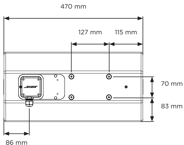
背面図
