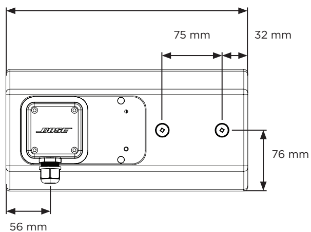
背面図
