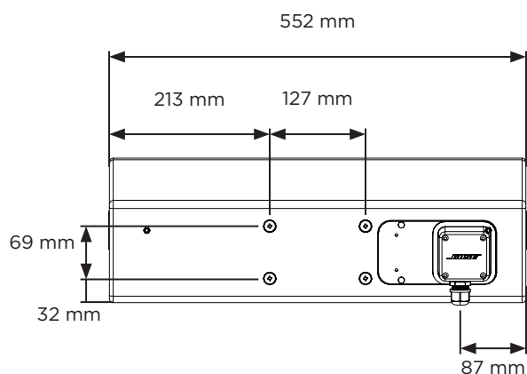
背面
