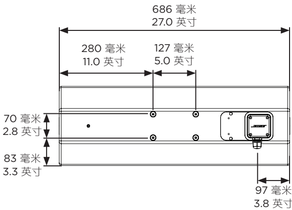
后视图
