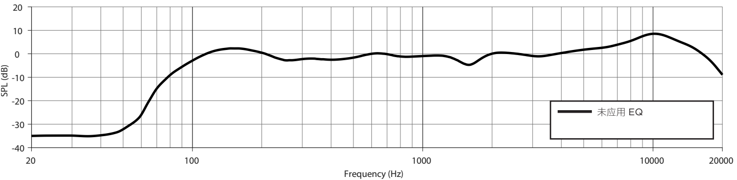
AMU208 频率响应
