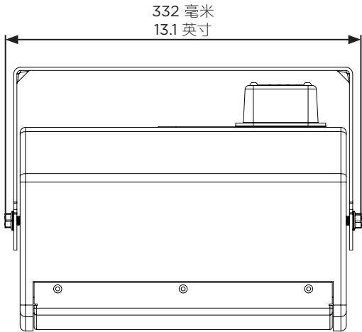
顶视图
