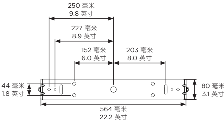
后视图
