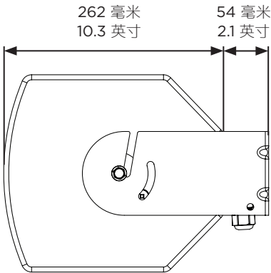
后视图
