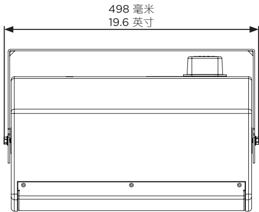
顶视图
