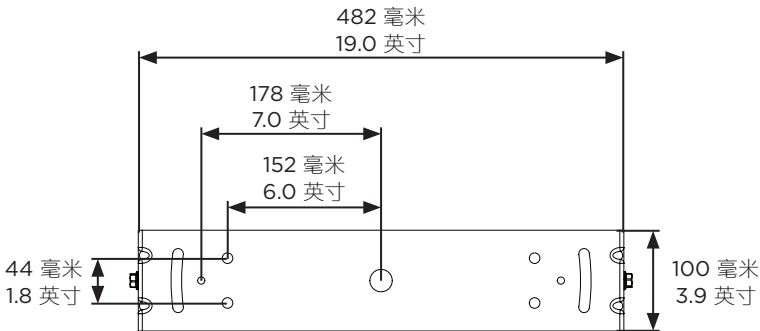
后视图
