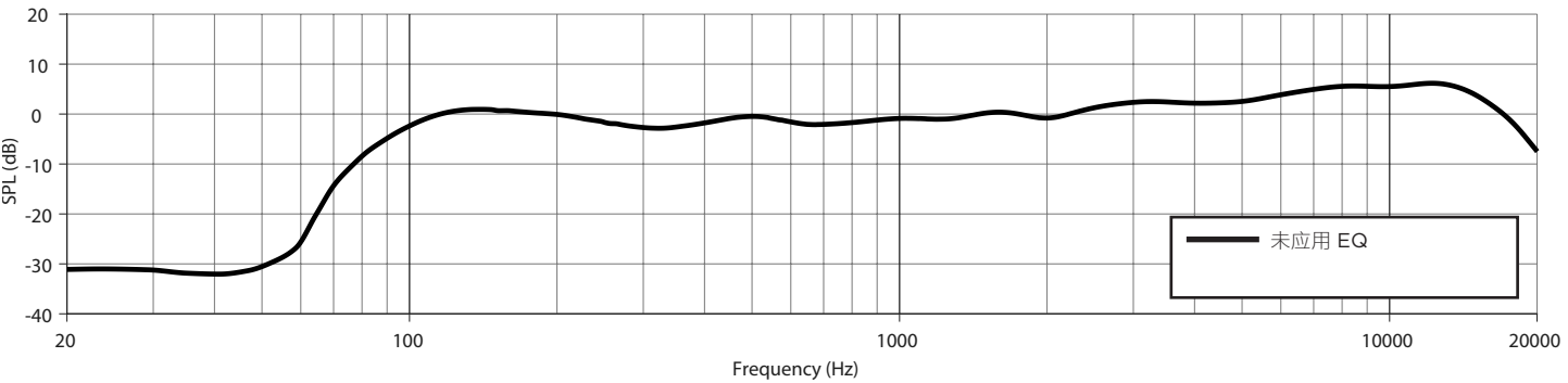
AMU206 频率响应
