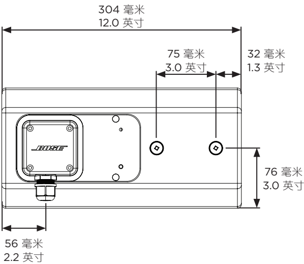
后视图
