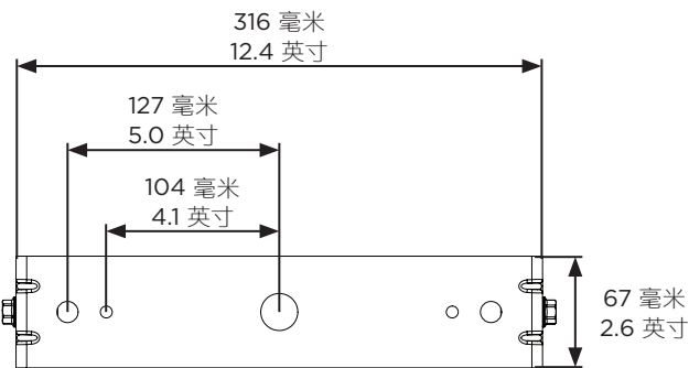
后视图
