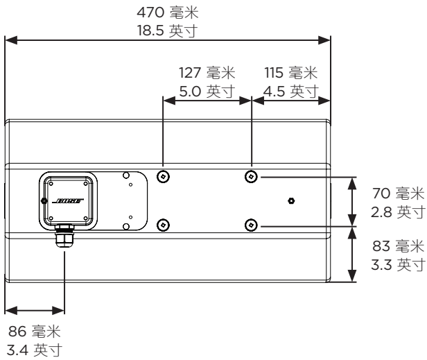
后视图
