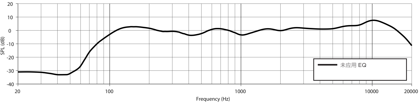
AMU108 频率响应
