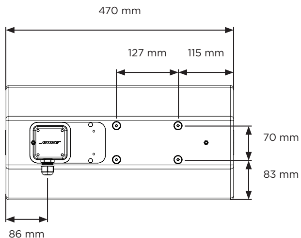
背面図
