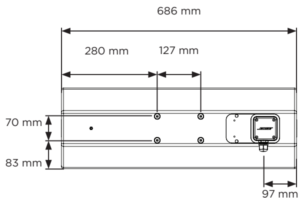
背面
