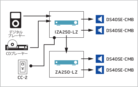
システム系統図
