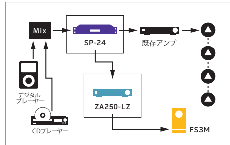
システム系統図 (AFTER)
