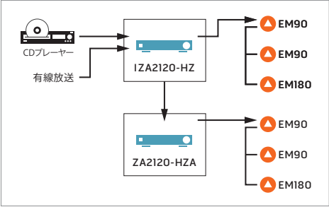
システム系統図
