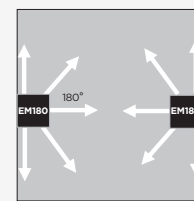
Room Placement Top View EM180は、水平180°の指向角を持ち、壁側のコーナー以外の天井に設置して使用します。
