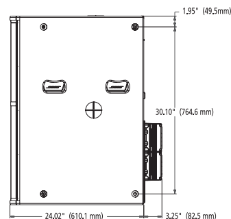
侧视图 (不含面网)
