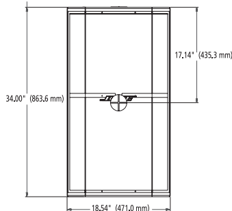
正视图 (含面网)
