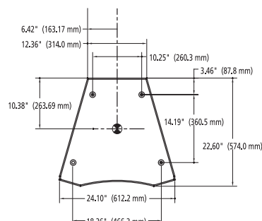
顶部/底部视图 (不含面网)
