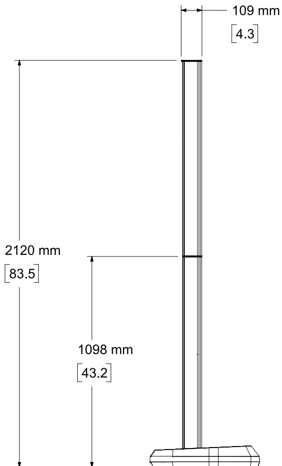
Seitenansicht
