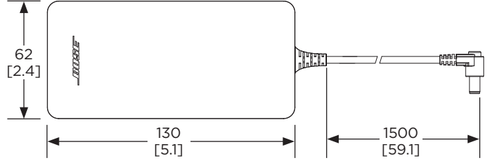
顶视图 电源
