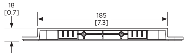
后视图 桌面支架
