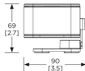
右视图 桌面安装 两侧尺寸
