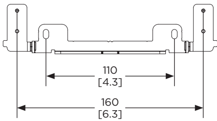
正视图 墙面安装支架
