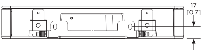
后视图 墙面安装
