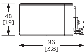
右视图 墙面安装 两侧尺寸
