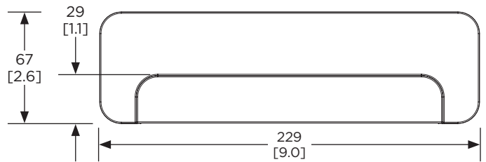
顶视图 桌面支架
