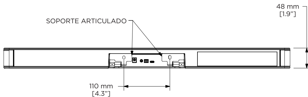
Vista trasera
