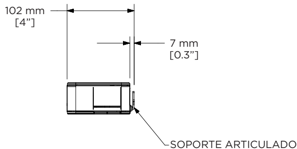
Vista derecha
